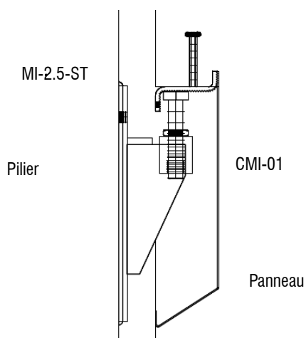
Montage du CMI-01 avec MI-2.5-ST
